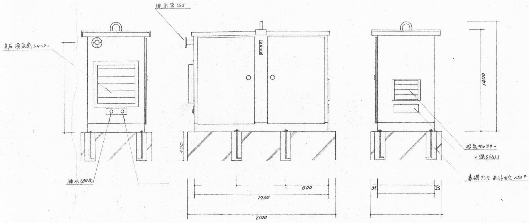
自家発電機 外観図
